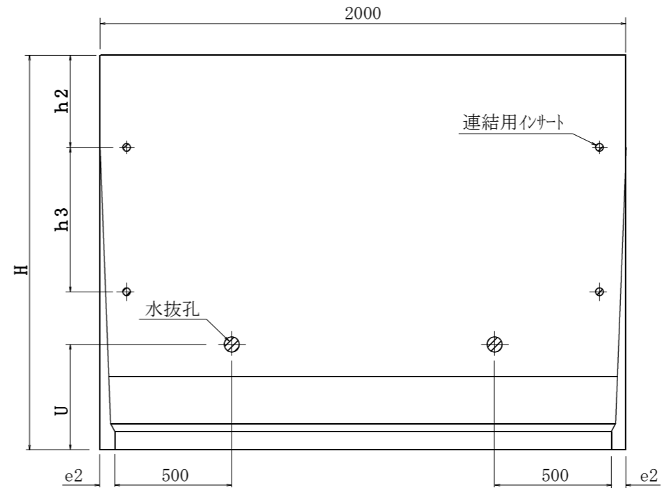
背面図
