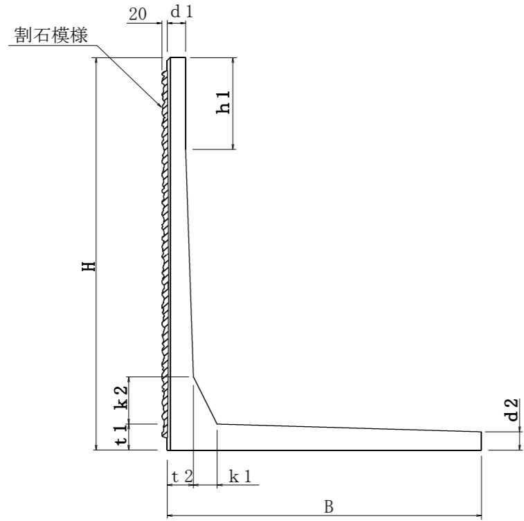
断面図
