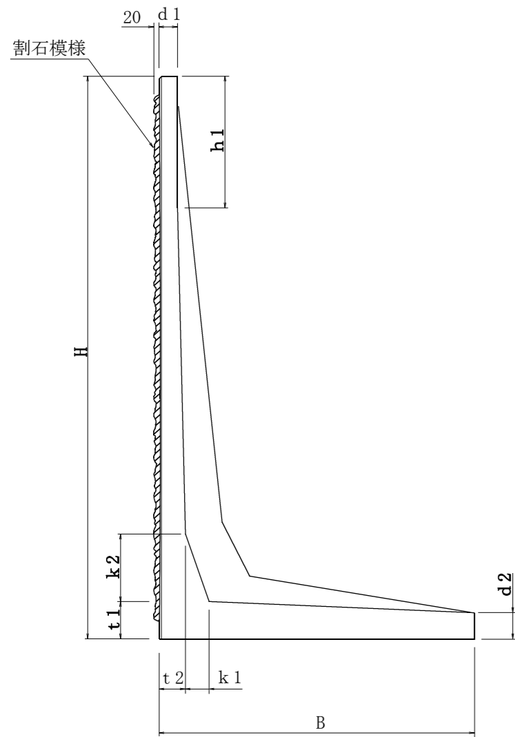
断面図
