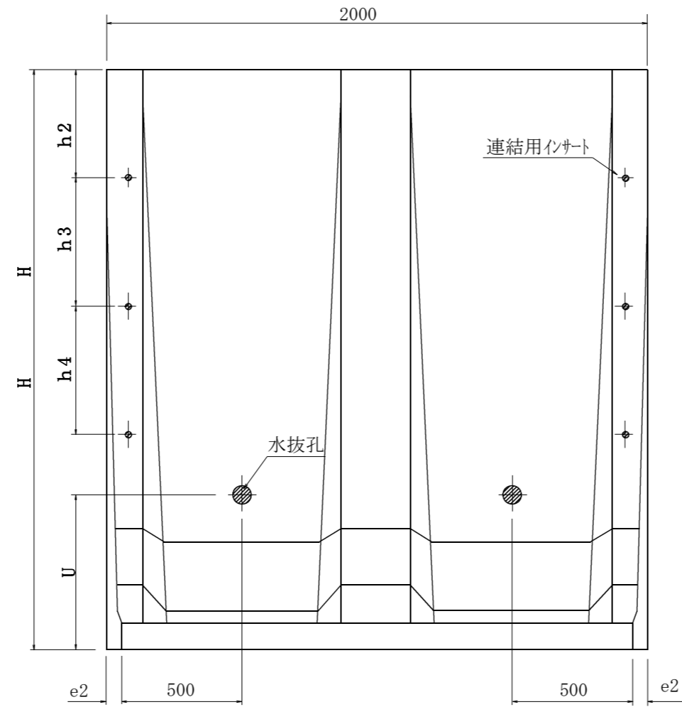
背面図
